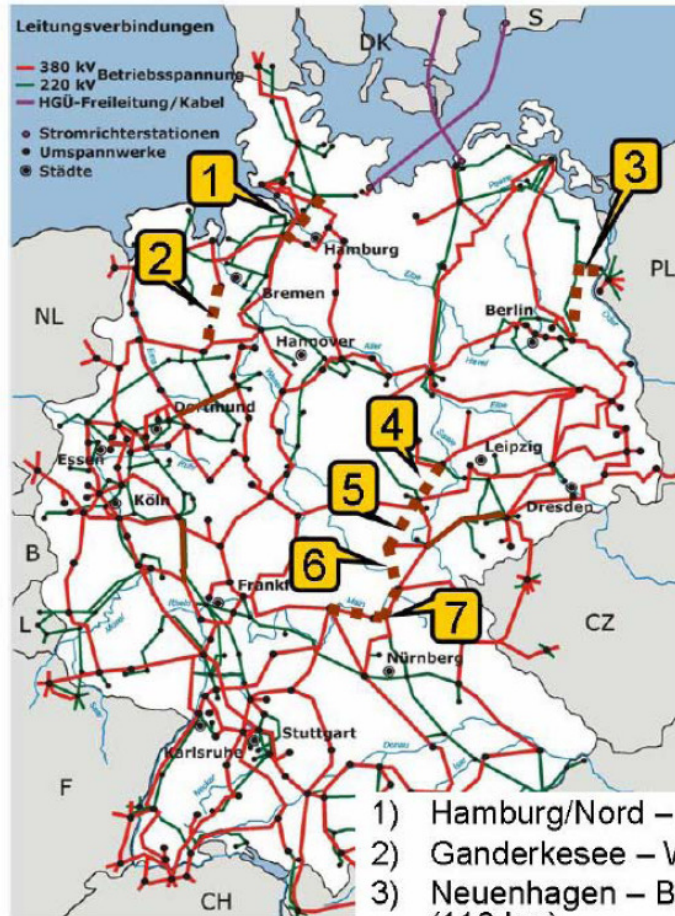
Abbildung 2: Netzverstärkungen und Netzausbau im Höchstspannungsübertragungsnetz zwischen 2007 und 2010
